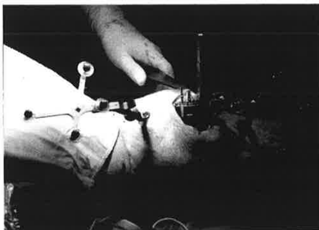
Abb. 3: Sägeblockpositionierung für die distale Femurresektion
